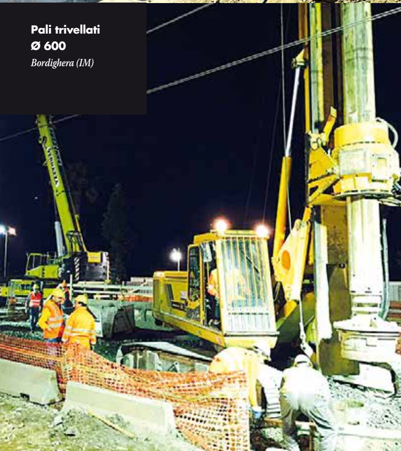
GEAX DTC 50 Fase del getto Sant'Elpidio a Mare (FM)
